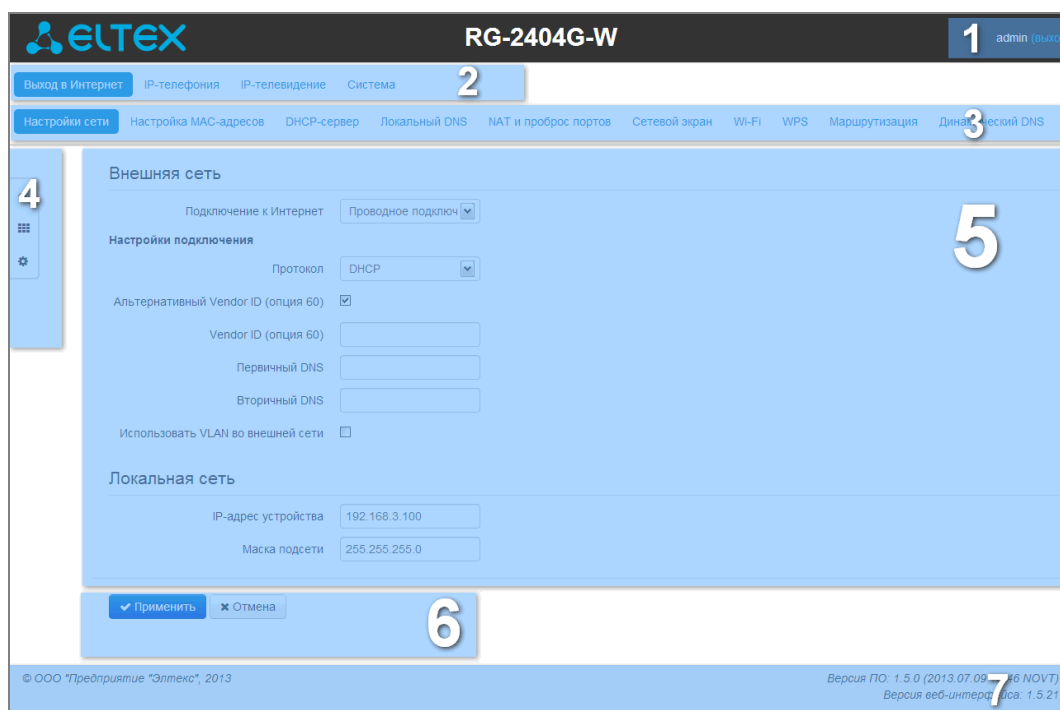
Рисунок 8 – Элементы навигации Web-конфигуратора
