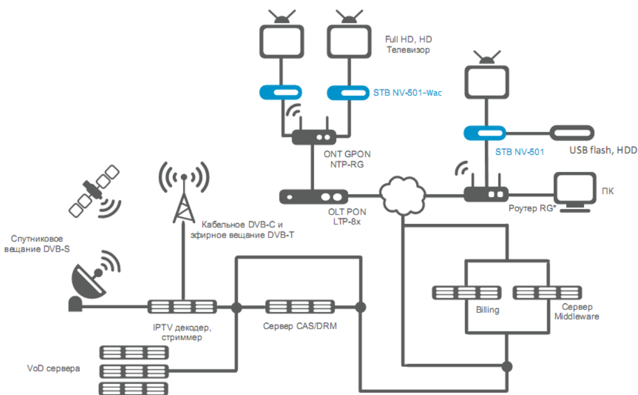
Рисунок 1 – Схема применения
