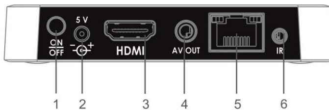
Рисунок 3– Внешний вид задней панели устройства
