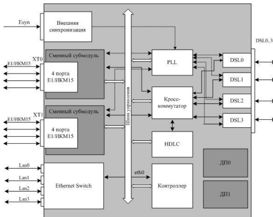
Рисунок 2 – Функциональная схема
