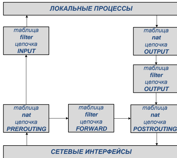
Рисунок 5 – Последовательность обработки пакетов и цепочки правил
