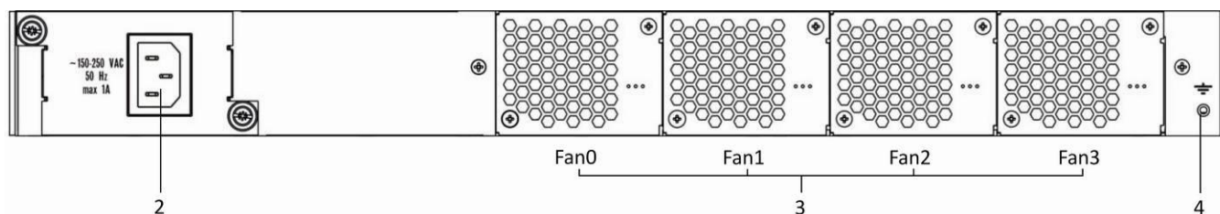
Рисунок 5 – Задняя панель станционного терминала LTE -8X, LTE-2X (AC)
