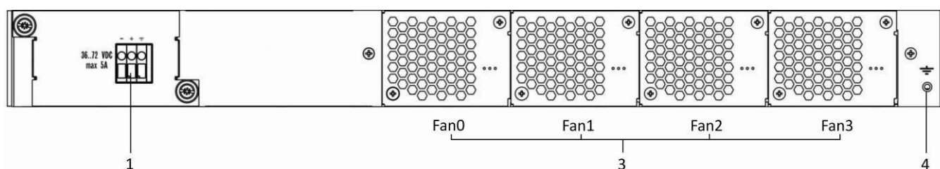
Рисунок 4 – Задняя панель станционного терминала LTE -8X, LTE-2X (DC)
