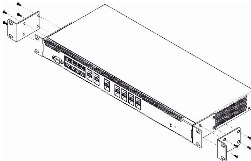
Рисунок 7 – Крепление кронштейнов
