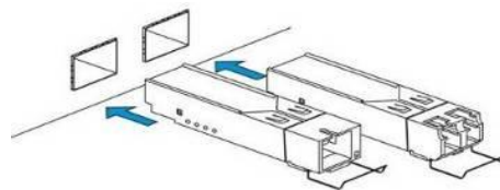
Рисунок 10 – Установка SFP-трансиверов
