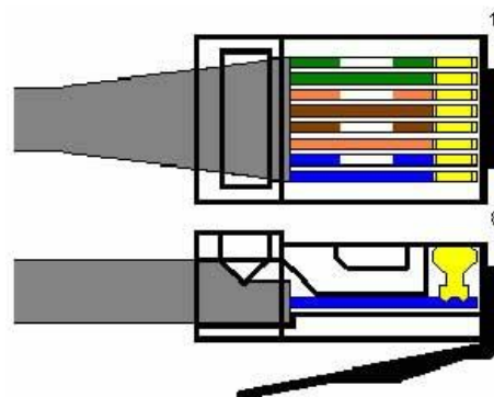
Разъем RJ-45
