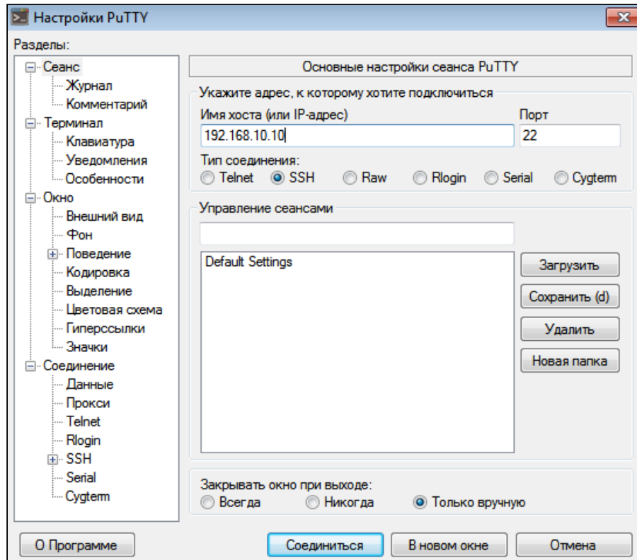
Рисунок 2 – Запуск SSH-клиента
