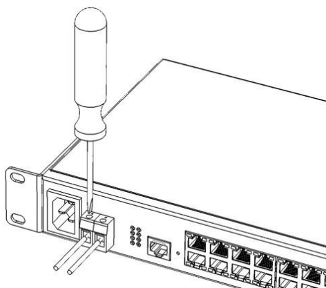
Рисунок 24 – Подключение АКБ к устройству
