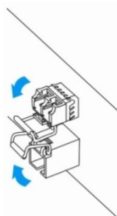
Рисунок 27 – Открытие защелки SFP-трансиверов
