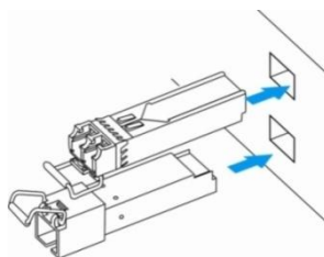
Рисунок 25 – Установка SFP-трансиверов
