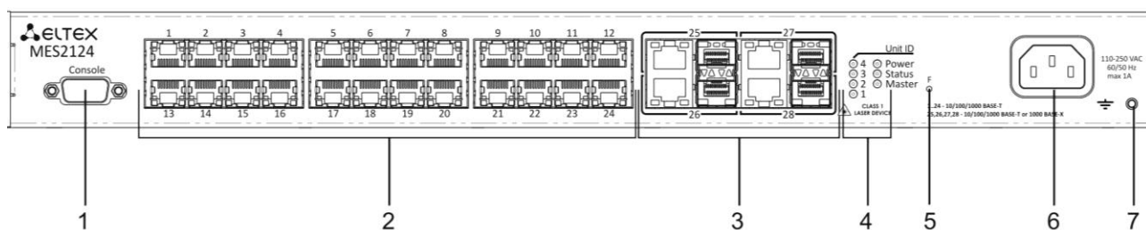
Рисунок 3 – MES2124, передняя панель
