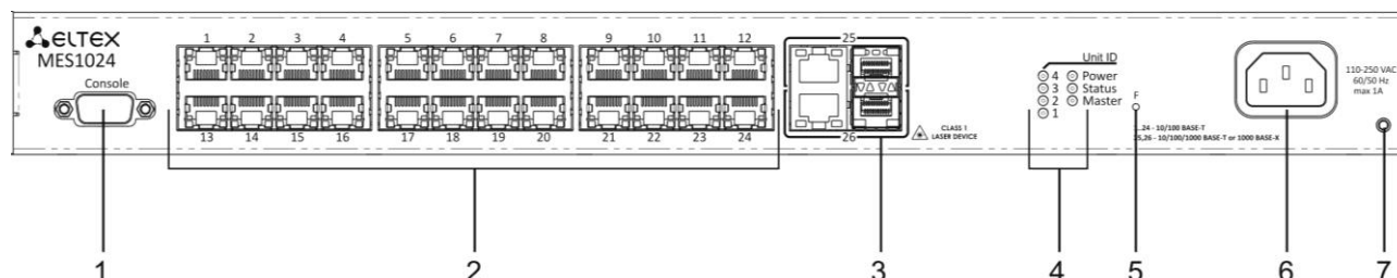
Рисунок 1 – MES1024, передняя панель
