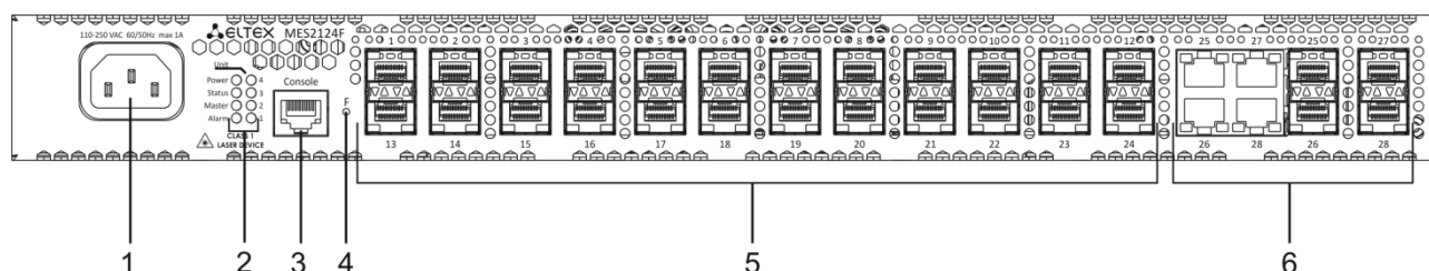
Рисунок 15 – MES2124F, передняя панель
