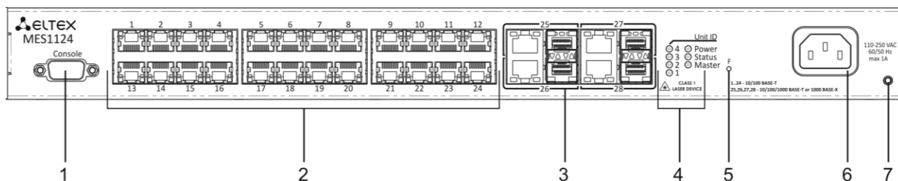
Рисунок 2 – MES1124, передняя панель
