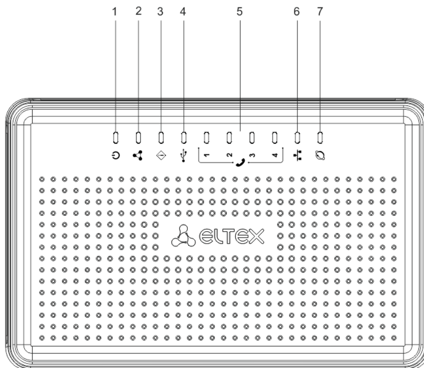
Рисунок 4 – Внешний вид верхней панели TAU-4M.IP
