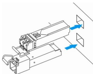
Рисунок 43 – Установка SFP-трансиверов
