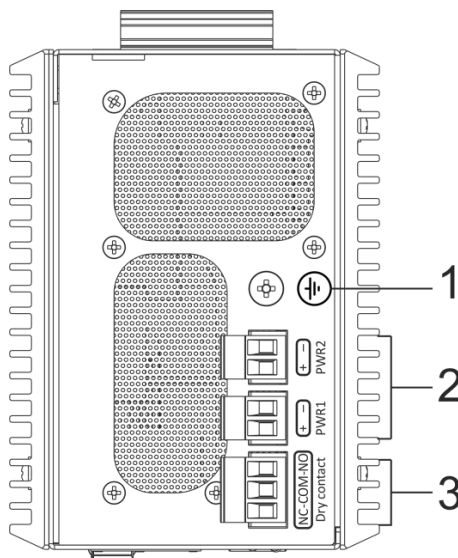
Рисунок 32 – Верхняя панель MES3508 и MES3508P
