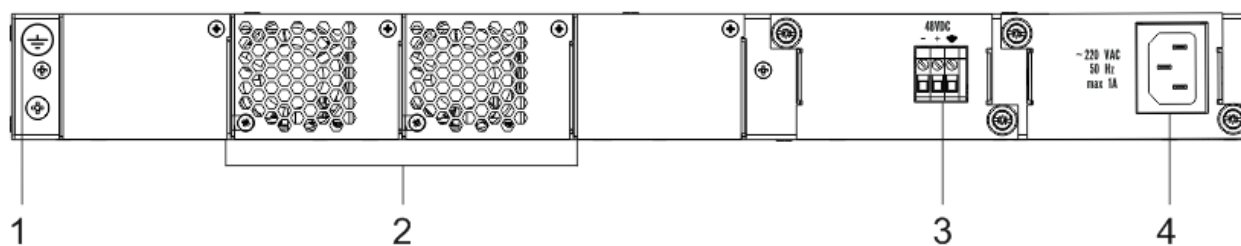
Рисунок 25 – Задняя панель MES3308F
