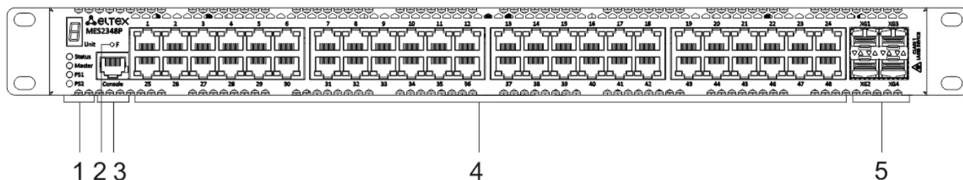
Рисунок 9 – Передняя панель MES2348P
