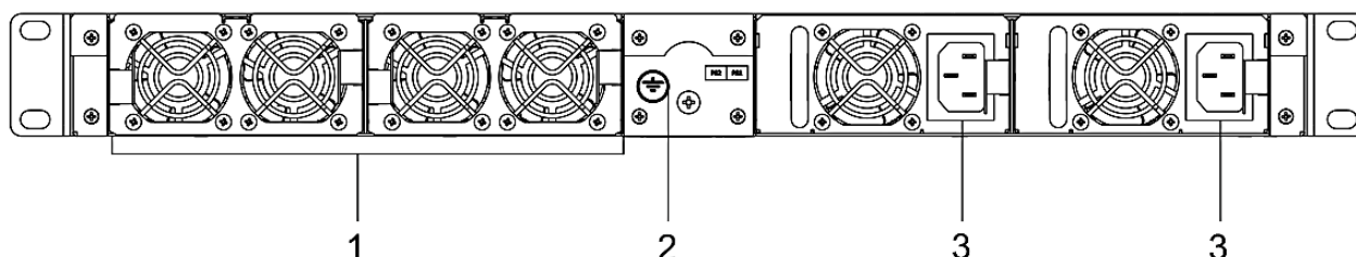
Рисунок 30 – Задняя панель MES2348P
