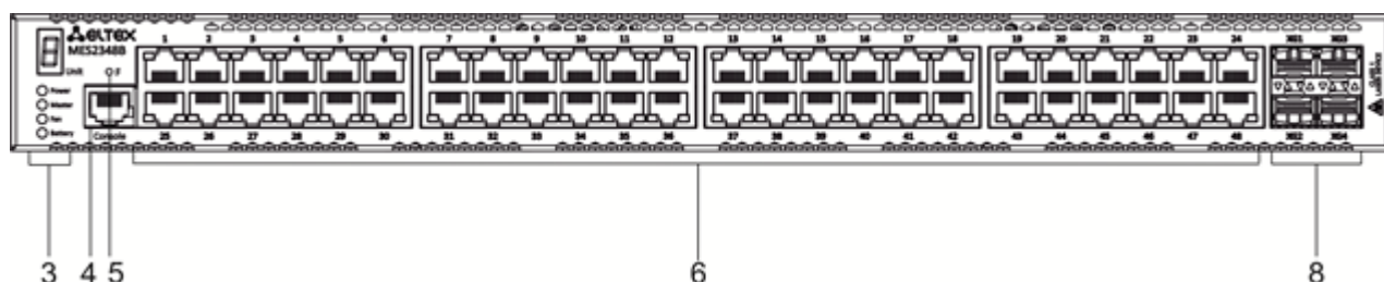
Рисунок 13 – MES2348B, передняя панель
