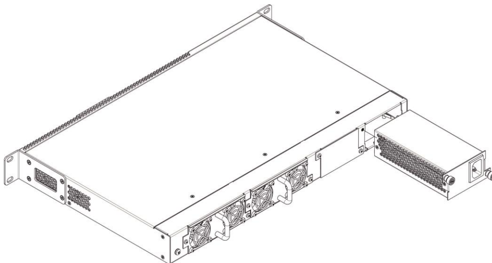
Рисунок 41 – Установка модулей питания
