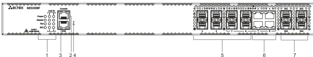
Рисунок 5 – Передняя панель MES3308F
