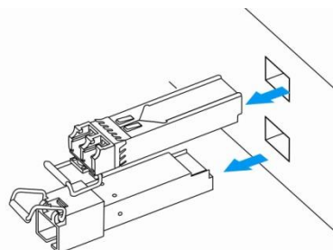
Рисунок 46 – Извлечение SFP-трансиверов
