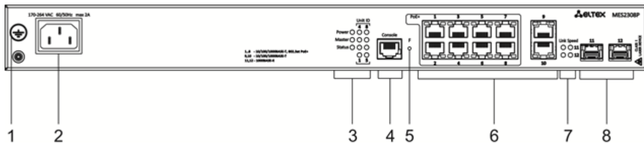
Рисунок 17 – Передняя панель MES2308P
