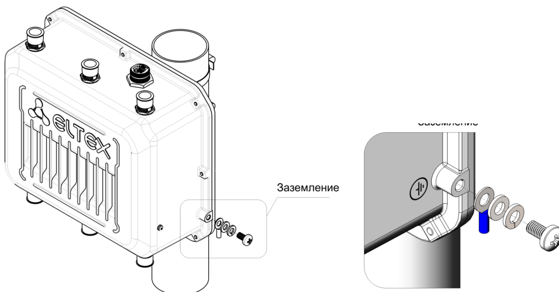
Рисунок 11 – Схема заземления устройства
