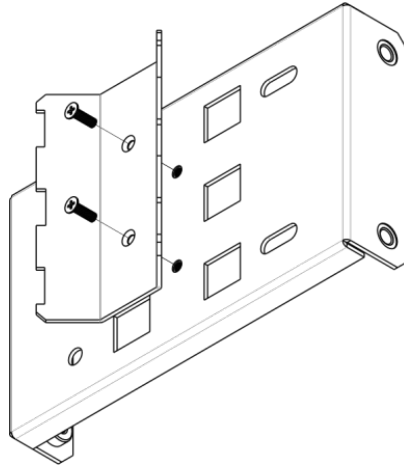
Рисунок 5 – Кронштейн для крепления на трубостойку
