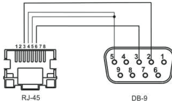
Рисунок 14 – Распайка консольного кабеля RJ45-DB9
