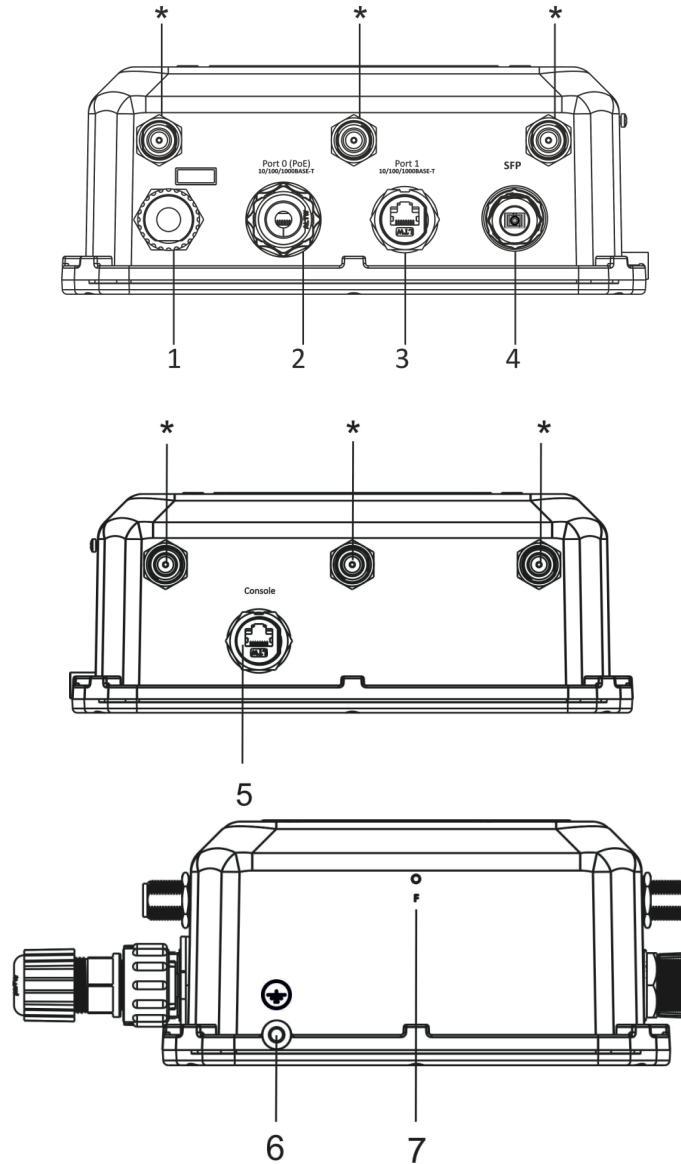
Рисунок 1 – Внешний вид боковых панелей WOP-12ac-LR
