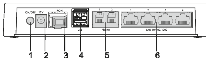
Рисунок 6 – Внешний вид задней панели NTU-RG RG-1422G-Wac
