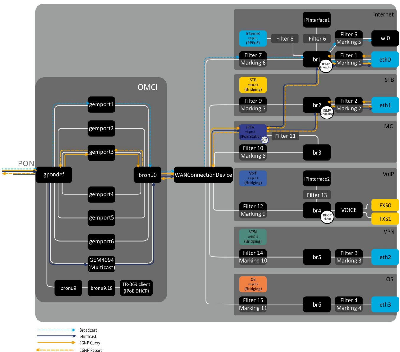
Рисунок 9 – Архитектура устройства, сконфигурированного для предоставления услуг Triple Play по модели 1
