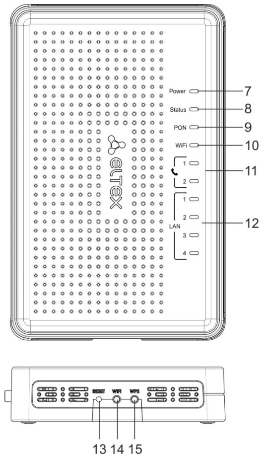
Рисунок 5 – Внешний вид боковой и верхней панели NTU-RG-1402G-W
