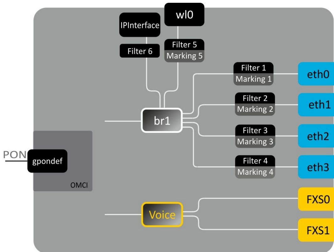
Рисунок 8 – Логическая архитектура устройства с заводской конфигурацией
