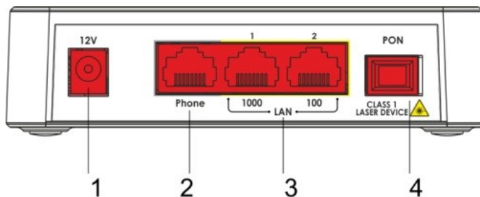
Рисунок 2 – Внешний вид задней панели NTU-2V
