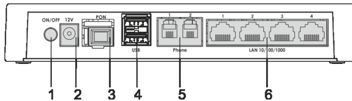
Рисунок 4 – Внешний вид задней панели NTU-RG-1402G-W
