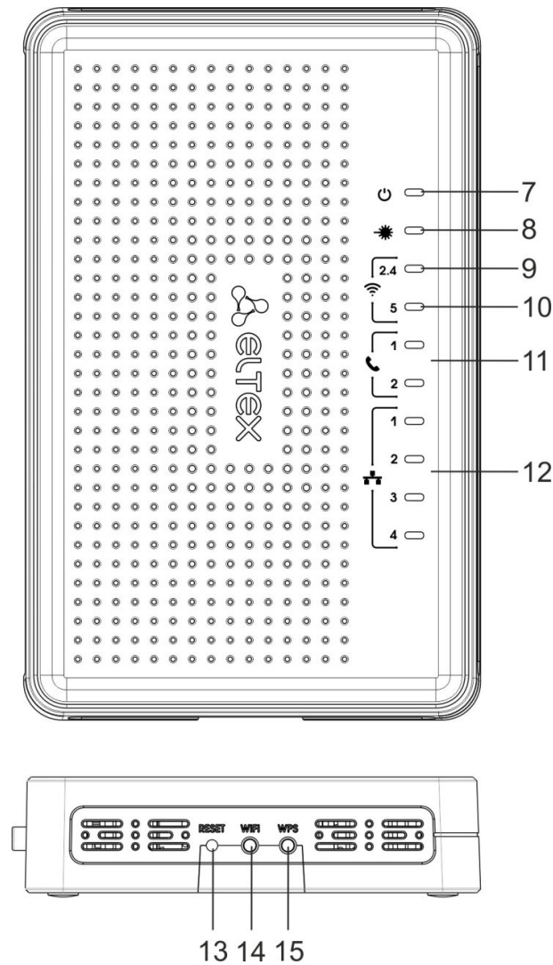
Рисунок 7 – Внешний вид боковой и верхней панели NTU-RG
