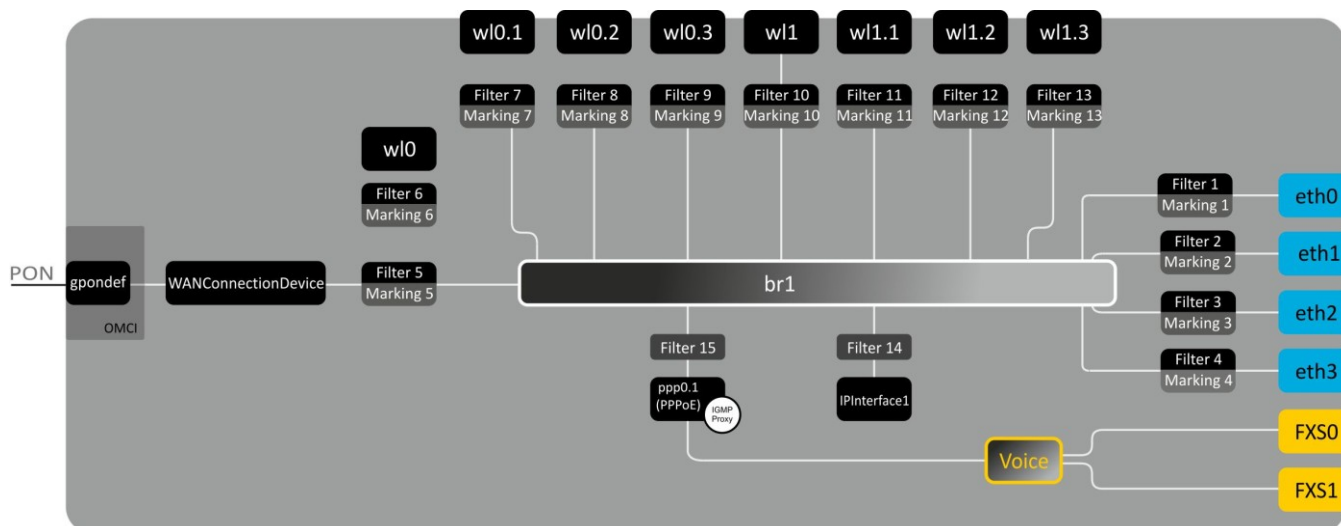
Рисунок 11 – Логическая архитектура устройства с заводской конфигурацией
