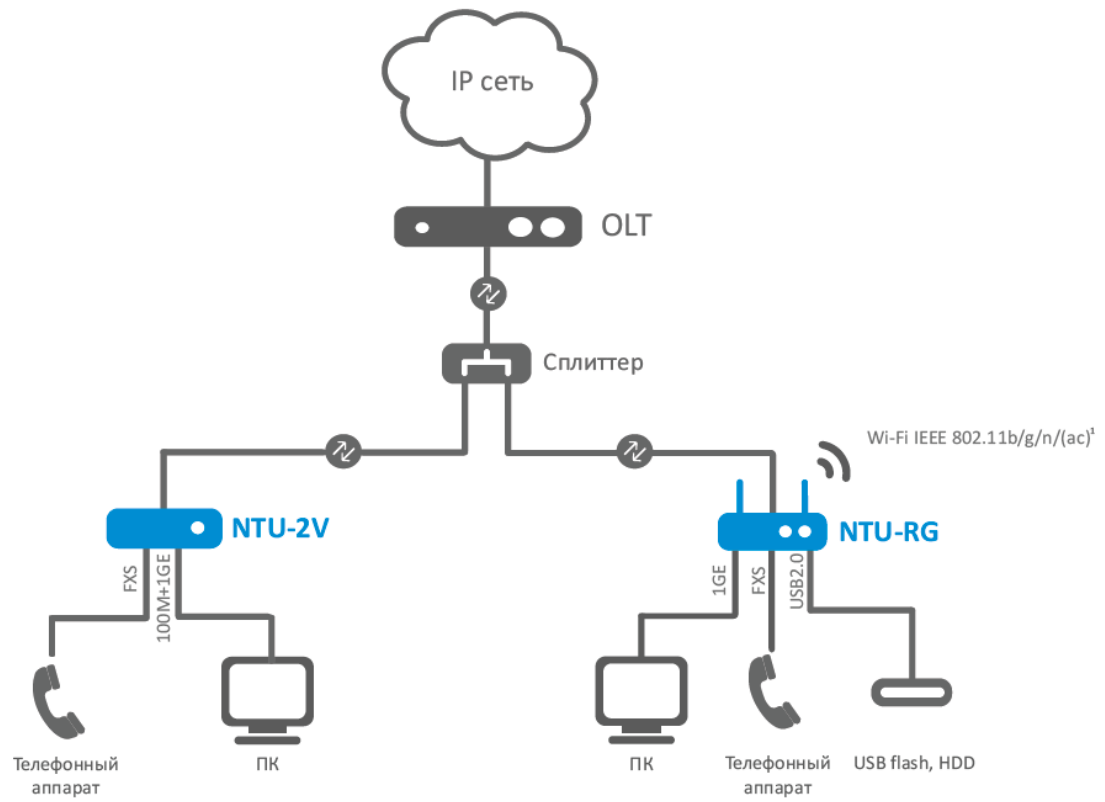
Рисунок 1– Схема применения NTU-2, NTU-RG-1402G-W
