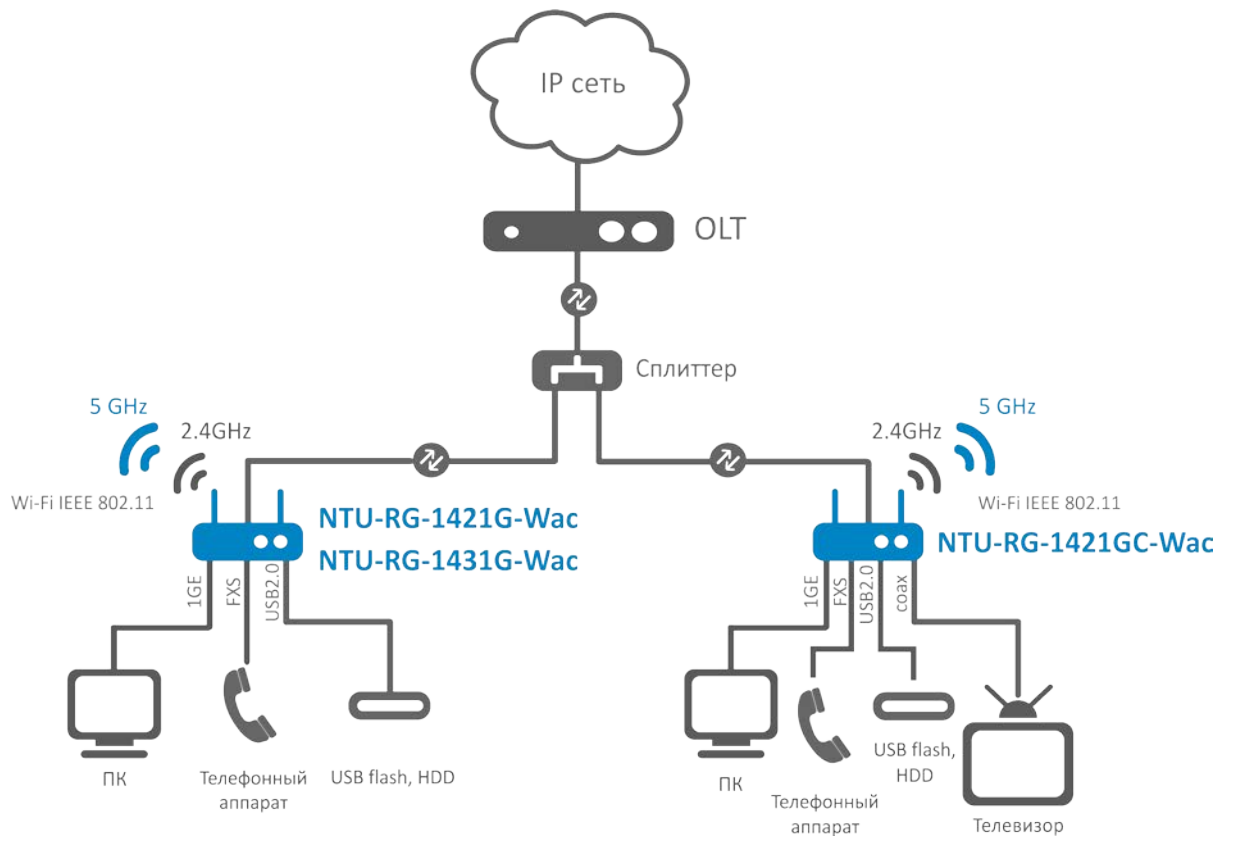
Рисунок 1 – Схема применения NTU-RG-1421G-Wac, NTU-RG-1431G-Wac, NTU-RG-1421GC-Wac
