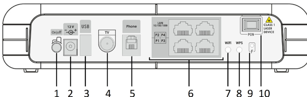
Рисунок 4 – Внешний вид задней панели NTU-RG-1421GC-Wac
