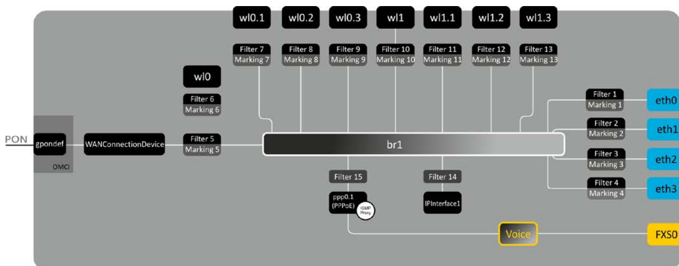
Рисунок 6 – Логическая архитектура устройства с заводской конфигурацией
