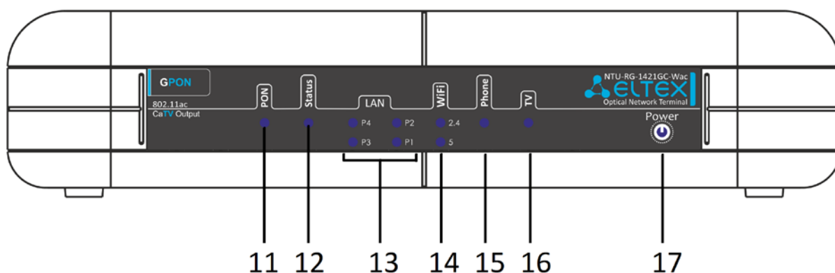
Рисунок 5 – Внешний вид передней панели NTU-RG-1421GC-Wac
