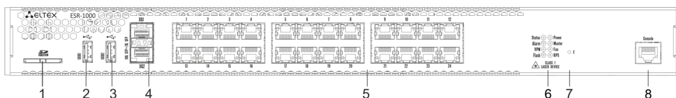
Рисунок 2.6 – Передняя панель ESR-1000
