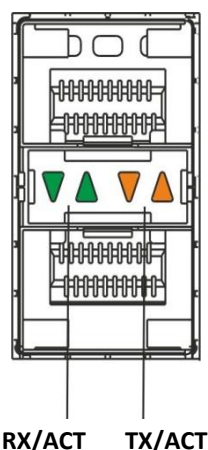
Рисунок 2.27 – Расположение индикаторов оптических интерфейсов
