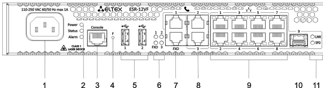
Рисунок 2.15 – Передняя панель ESR-12VF, ESR-14VF
