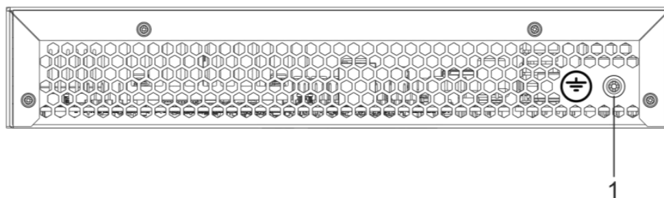
Рисунок 2.16 – Задняя панель ESR-12VF, ESR-14VF
