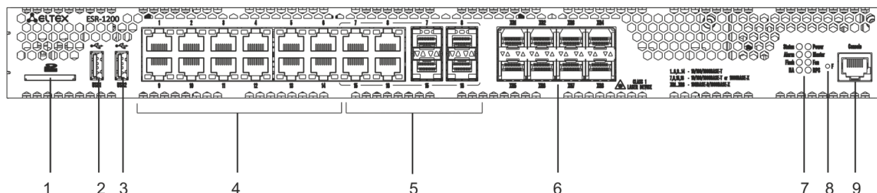
Рисунок 2.5 – Передняя панель ESR-1200
