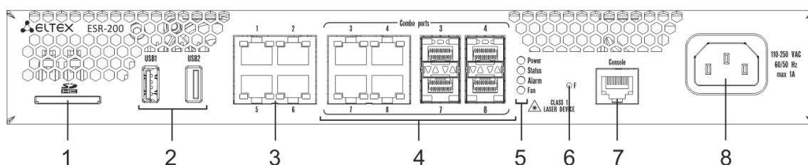
Рисунок 2.11 – Передняя панель ESR-200
