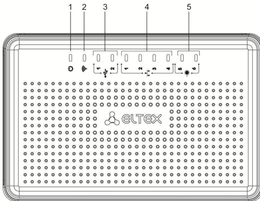
Рисунок 2.25 – Верхняя панель маршрутизатора ESR-10
