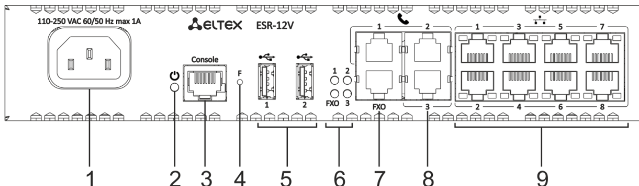
Рисунок 2.19 – Передняя панель ESR-12V
