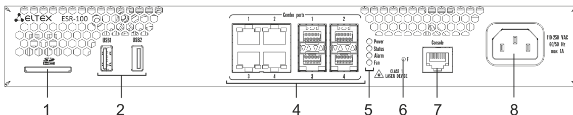
Рисунок 2.10 – Передняя панель ESR-100
