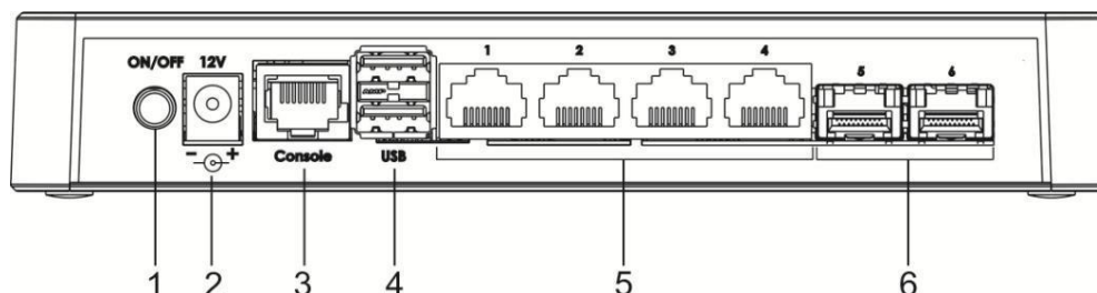
Рисунок 2.23 – Задняя панель ESR-10
