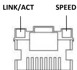
Рисунок 2.26 – Расположение индикаторов разъема RJ-45
