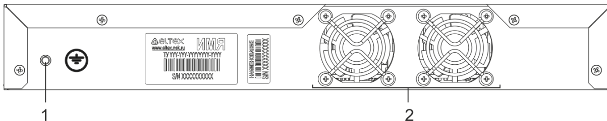
Рисунок 2.12 – ESR-100, ESR-200 задняя панель
