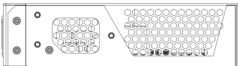
Рисунок 2.18 – Правая панель ESR-12VF, ESR-14VF
