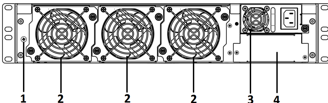
Рисунок 2.2 – Задняя панель ESR-1700
