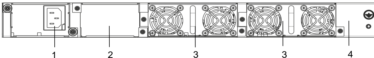
Рисунок 2.7 – Задняя панель ESR-1000, ESR-1200
