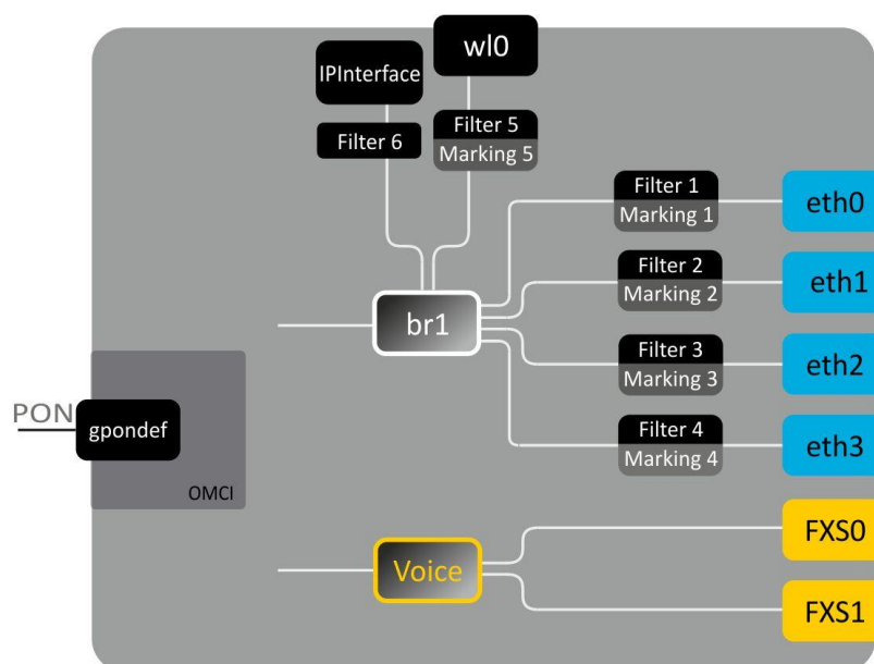
Рисунок 12 – Логическая архитектура устройства с заводской конфигурацией на примере NTP-RG ревизии С (rev.C)
