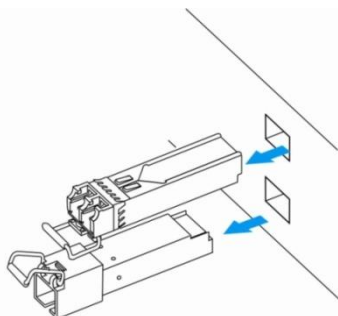
Рисунок 28 – Извлечение SFP-трансиверов
