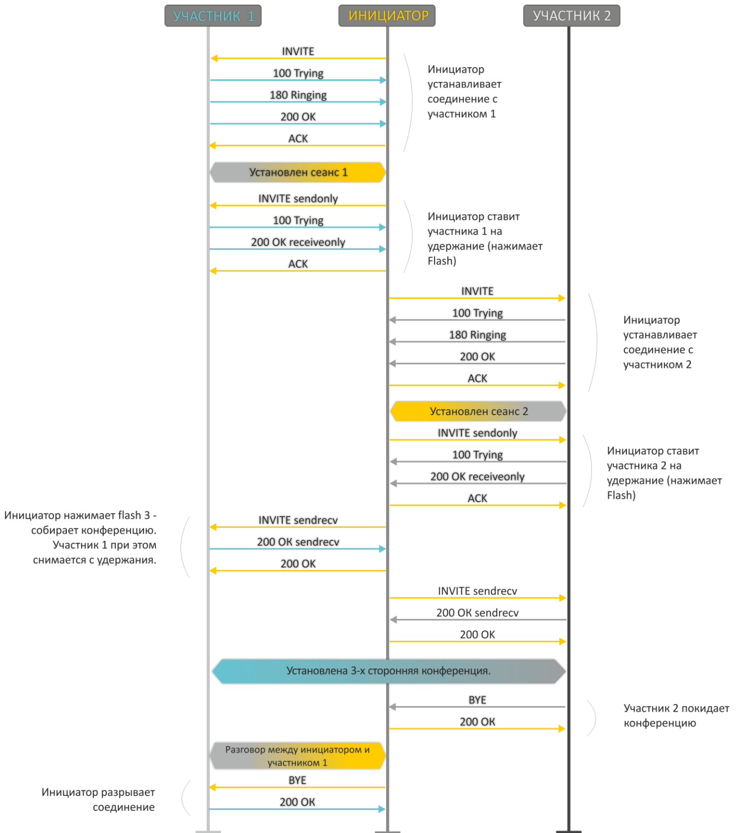
Рисунок 12 – Алгоритм выполнения услуги «Трёхсторонняя конференция» («3-way conference») локально на устройстве по протоколу SIP
