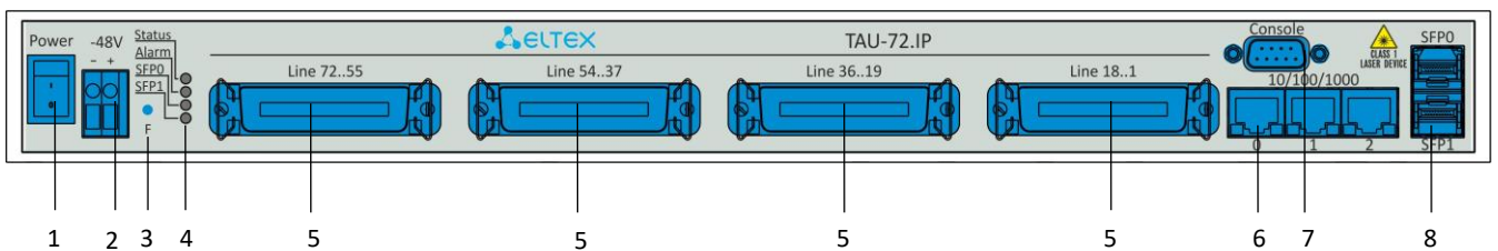
Рисунок 4в – Внешний вид передней панели TAU-72.IP v4.0 и rev.B с питанием от сети постоянного тока
