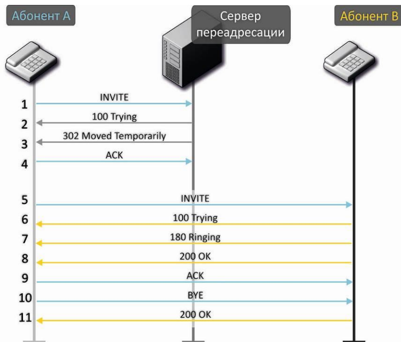
Рисунок 17 – Алгоритм вызова с участием сервера переадресации
