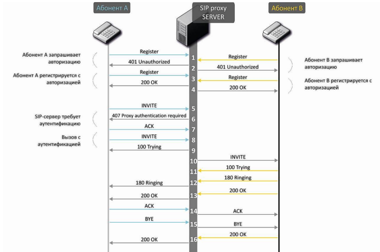
Рисунок 16 – Алгоритм вызова с участием SIP проху-сервера
