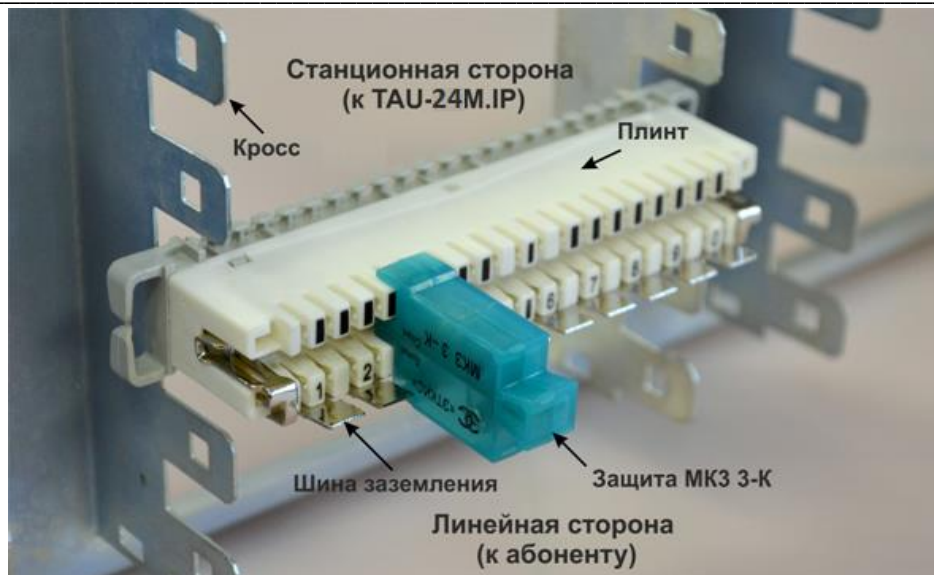
Рисунок 9 – Схема подключения
