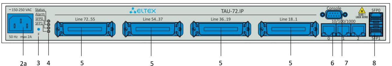
Рисунок 4г – Внешний вид передней панели TAU-72.IP v4.0 и rev.B с питанием от сети переменного тока
