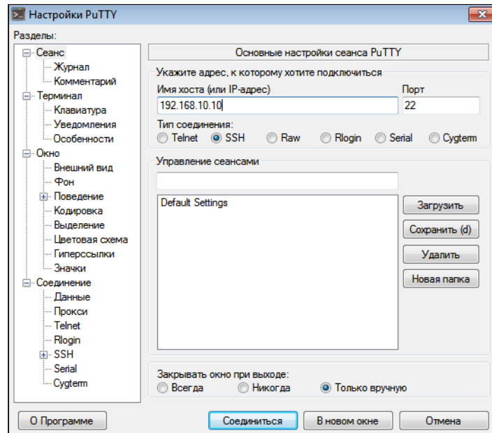
Рисунок 2 – Запуск SSH-клиента
