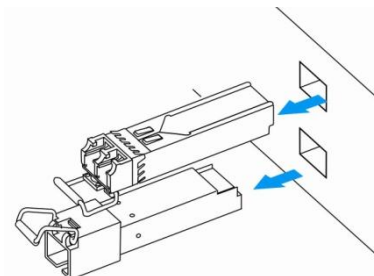
Рисунок 46 – Извлечение SFP-трансиверов
