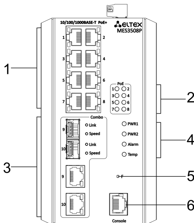
Рисунок 20 – Передняя панель MES3508P
