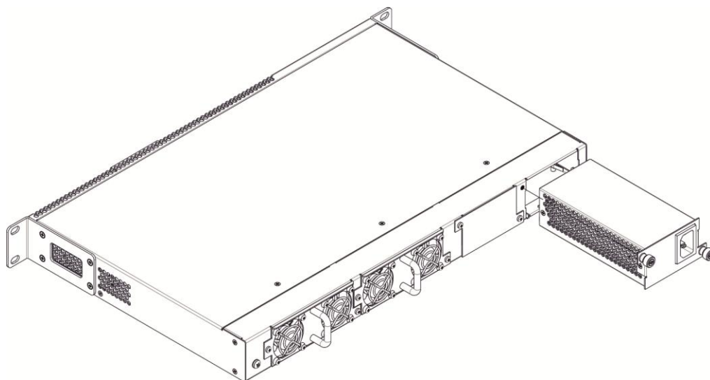
Рисунок 41 – Установка модулей питания
