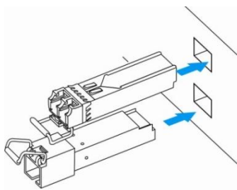
Рисунок 43 – Установка SFP-трансиверов
