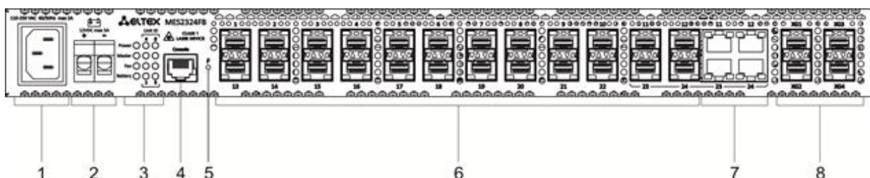
Рисунок 11 – MES2324FB, передняя панель
