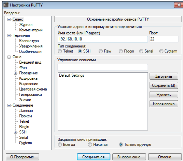
Рисунок 2 – Запуск SSH-клиента
