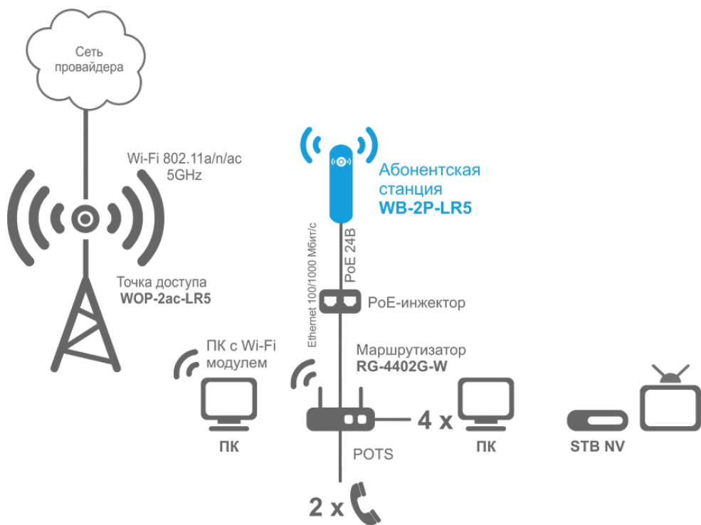
Функциональная схема использования WB-2P-LR5 с маршрутизатором
