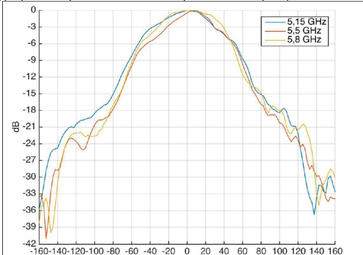
Диаграмма направленности антенны вертикальной поляризации в Е-плоскости:
