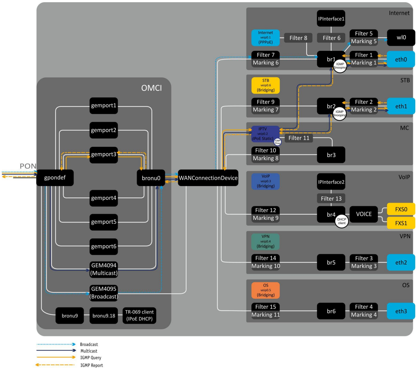
Рисунок 20 – Архитектура устройства, сконфигурированного для предоставления услуг Triple Play по модели 2
