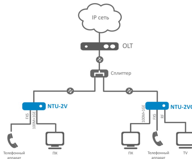
Рисунок 1 – Схема применения NTU-2V, NTU-2VC
