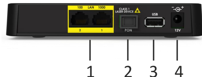
Рисунок 8 – Внешний вид задней панели NTU-2W
