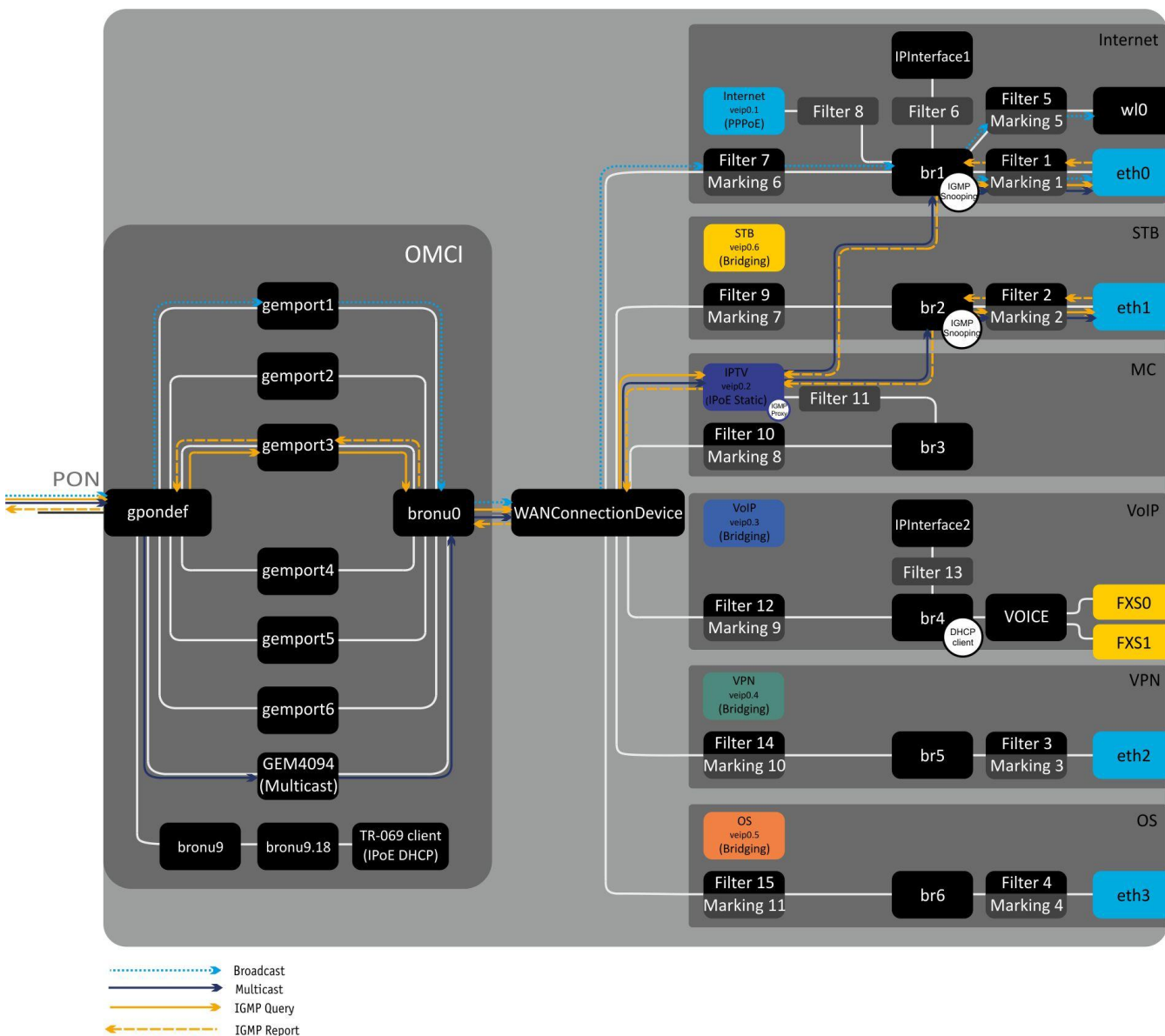
Рисунок 19 – Архитектура устройства, сконфигурированного для предоставления услуг Triple Play по модели 1
