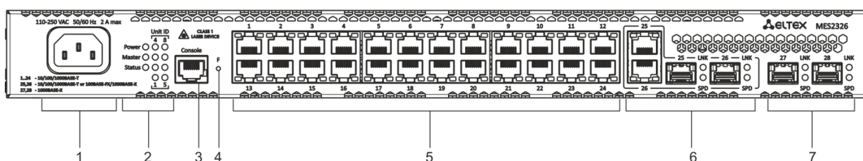
Рисунок 6 – Передняя панель MES2326
