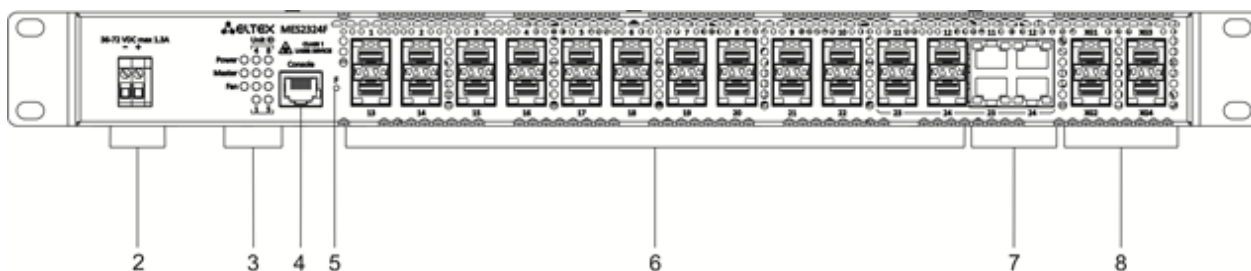
Рисунок 12 – MES2324F DC, передняя панель
