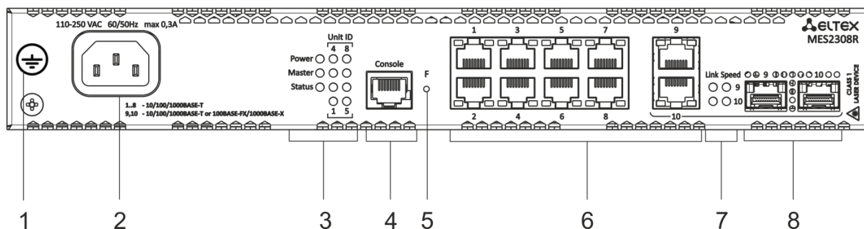
Рисунок 19 – Передняя панель MES2308R
