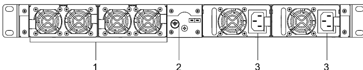
Рисунок 30 – Задняя панель MES2348P
