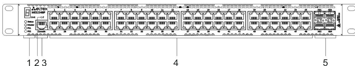
Рисунок 9 – Передняя панель MES2348P
