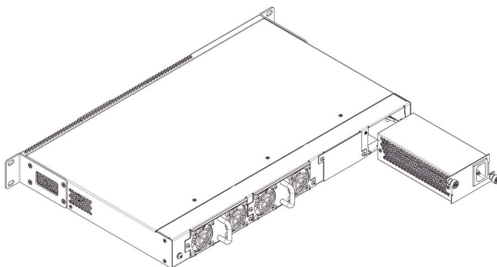
Рисунок 41 – Установка модулей питания
