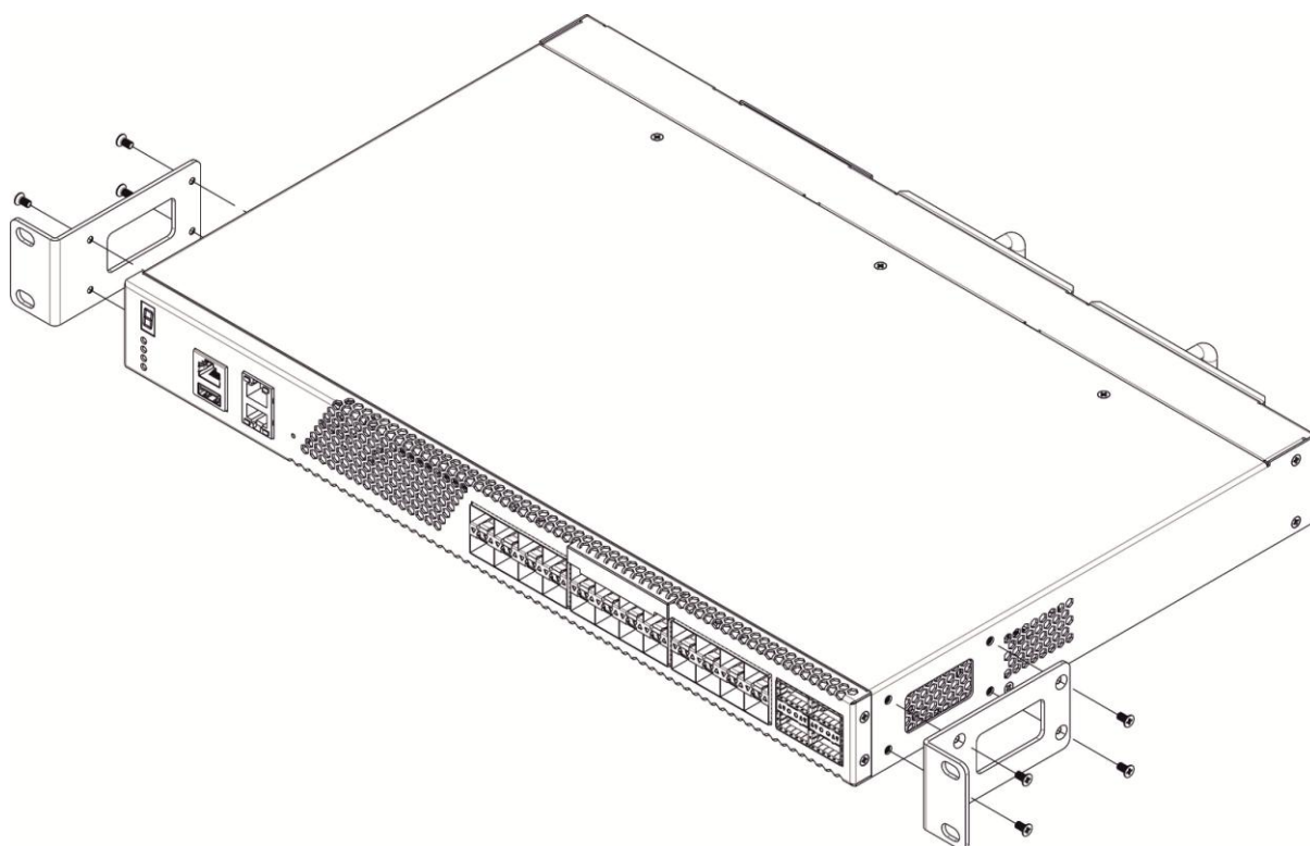
Рисунок 38 – Крепление кронштейнов
