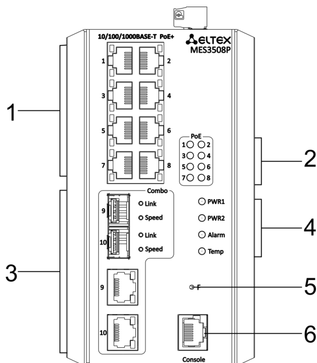
Рисунок 20 – Передняя панель MES3508P
