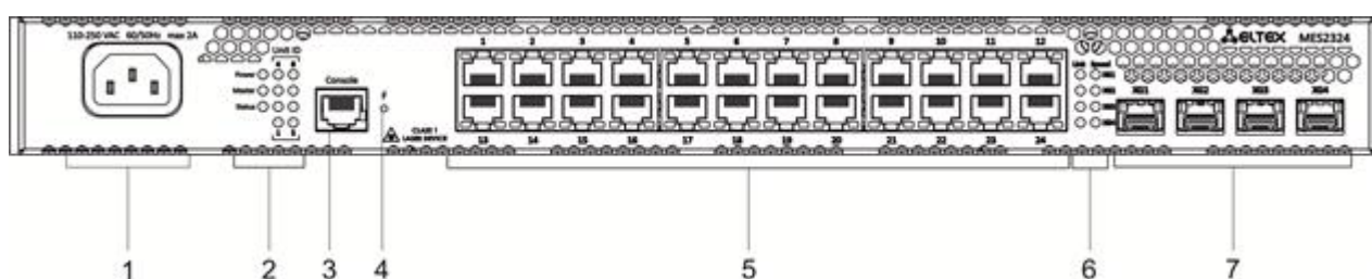
Рисунок 7 – Передняя панель MES2324
