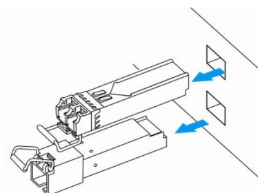
Рисунок 46 – Извлечение SFP-трансиверов
