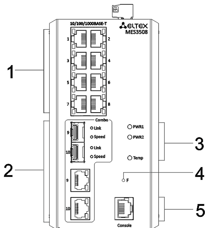
Рисунок 21 – Передняя панель MES3508
