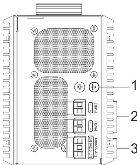
Рисунок 32 – Верхняя панель MES3508 и MES3508P
