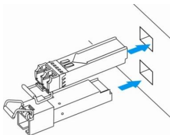
Рисунок 43 – Установка SFP-трансиверов
