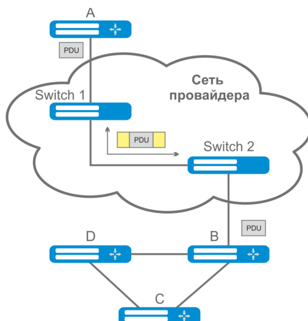
Рисунок 48 – Пример работы функции L2PT
