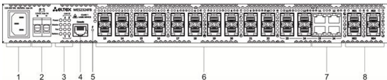
Рисунок 11 – MES2324FB, передняя панель
