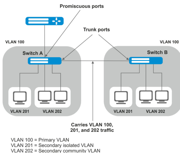
Рисунок 47 – Пример работы технологии Private VLAN
