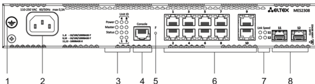
Рисунок 16 – Передняя панель MES2308
