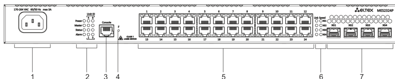
Рисунок 8 – Передняя панель MES2324P
