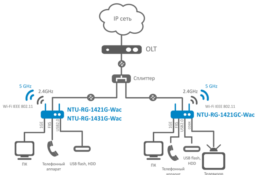
Рисунок 1 – Схема применения NTU-RG-1421G-Wac, NTU-RG-1431G-Wac, NTU-RG-1421GC-Wac
