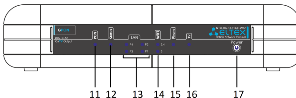
Рисунок 6 – Внешний вид передней панели NTU-RG-1421GC-Wac
