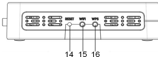
Рисунок 4 – Внешний вид боковой панели NTU-RG
