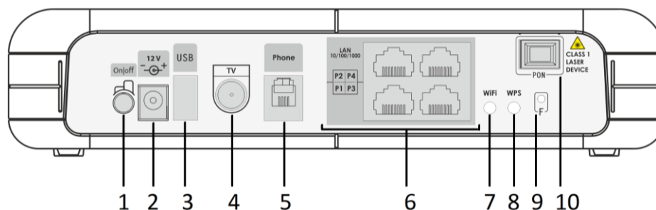
Рисунок 5 – Внешний вид задней панели NTU-RG-1421GC-Wac
