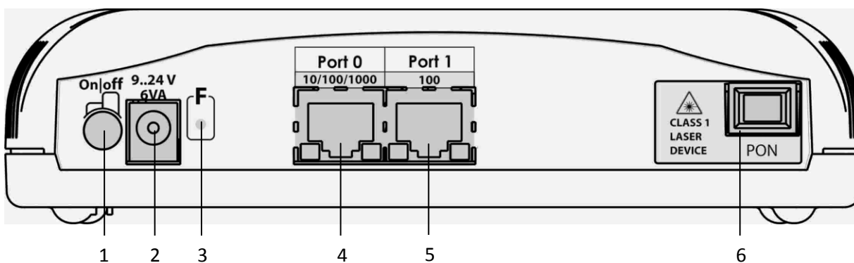
Рисунок 3 – Задняя панель абонентского терминала NTE-2
